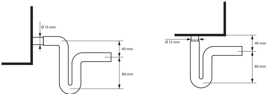
Мал. 17а. Монтаж сифона без зворотного клапана
