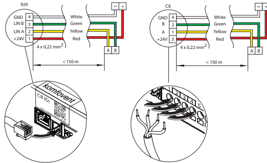
Мал. 22. Електрична схема дроту пульта
