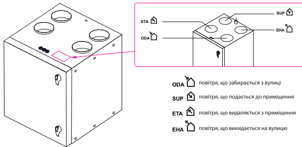
Мал. 14. Позначення повітроводів
