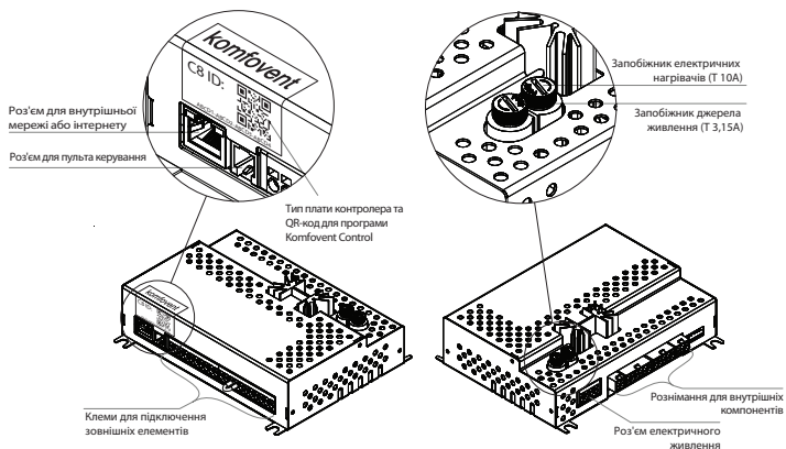
Мал. 18. Головна плата контролера C8
