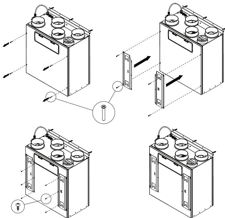
Fig. 11. Установка монтажных кронштейнів.
