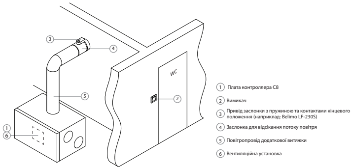
Мал. 15. Приклад монтажу повітроводу додаткової витяжки повітря
