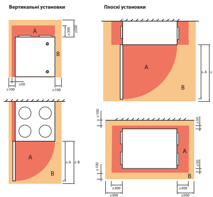
Мал. 5. Мінімальний простір для обслуговування установки
