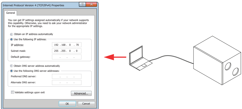
Мал. 25. Налаштування плати комп'ютерної мережі при підключенні безпосередньо до установки
