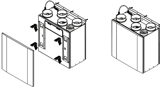
Fig. 12. Установка декоративної панелі
