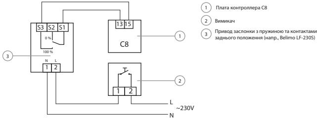
Мал. 21. Приклад включення вентиляційного режиму «Пріоритет», коли використовується додаткова витяжка повітря з моторизованою заслонкою (див. мал. 14)
