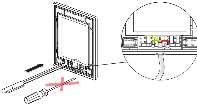
Мал. 23. Підключення кабелю до пульта
