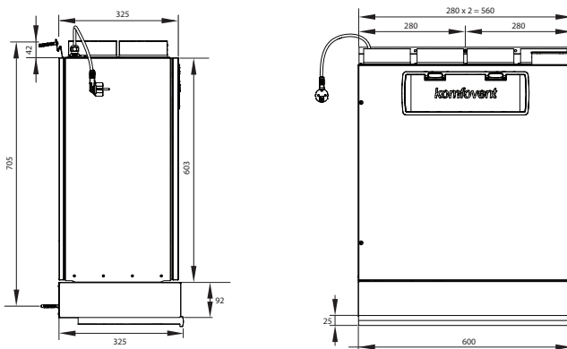
Fig. 9. Розміри з витяжним капюшоном 392-12
