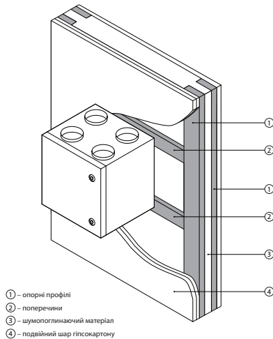
Рис. 7. Монтаж установки на гіпсокартонній перегородці
