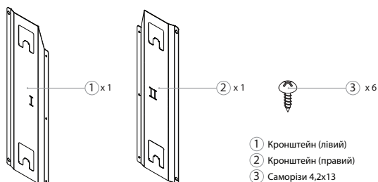
Fig. 10. Набір кріплень для монтажу панелей
