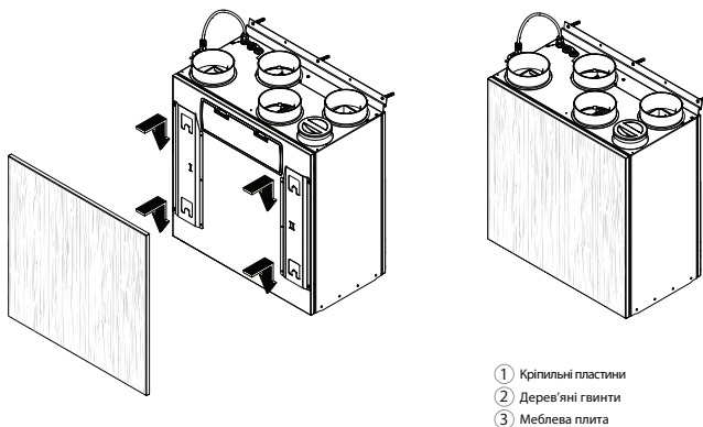
Fig. 13. Установка меблевої плити
