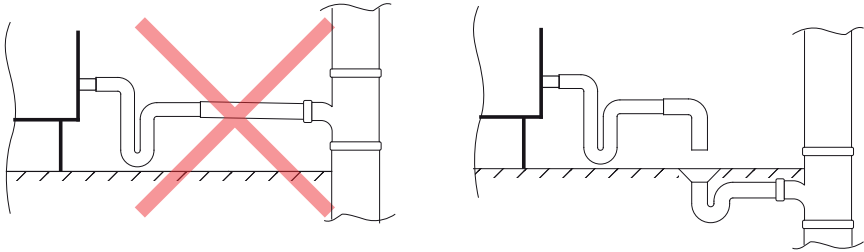
Мал. 176. Підключення відведення конденсату до каналізаційної системи
